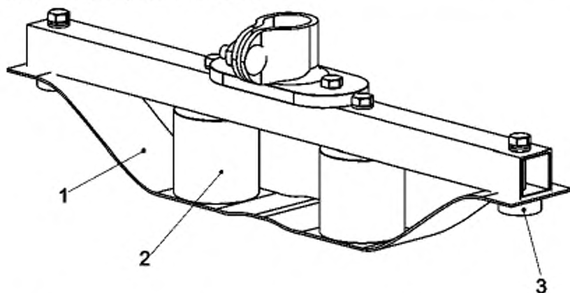
Рисунок 3 — Компоненты, включающие нагруженный контур, устройство измерения толщины подушки сиденья, средство поддержки RCLI на конце жесткого вала, позволяющее RCLI двигаться в направлении вперед на подушку сиденья в одной плоскости [см. 5.7, перечисления а) — d), и перечисления l) — q)]
