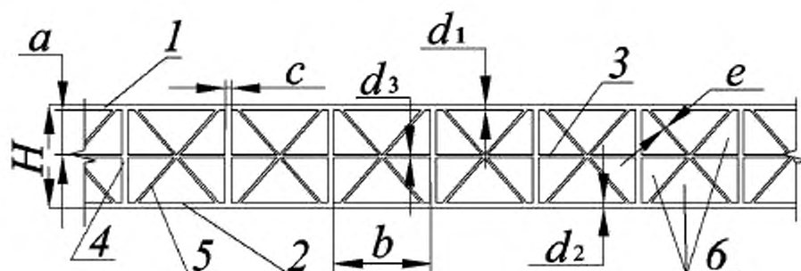
1 — внешний лицевой слой; 2 — внешний нелицевой слой; 3 — внутренний горизонтальный слой; 4 — вертикальные ребра жесткости; 5 — наклонные ребра жесткости; 6 — каналы; H — толщина панели; a — расстояние между горизонтальными слоями; b — расстояние между вертикальными ребрами жесткости; d_1 — толщина внешнего лицевого слоя; d_2 — толщина внешнего нелицевого слоя; d_3, d_4, \dots, d_n — толщина внутренних горизонтальных слоев; c — толщина вертикальных ребер жесткости; e — толщина наклонных ребер жесткости
