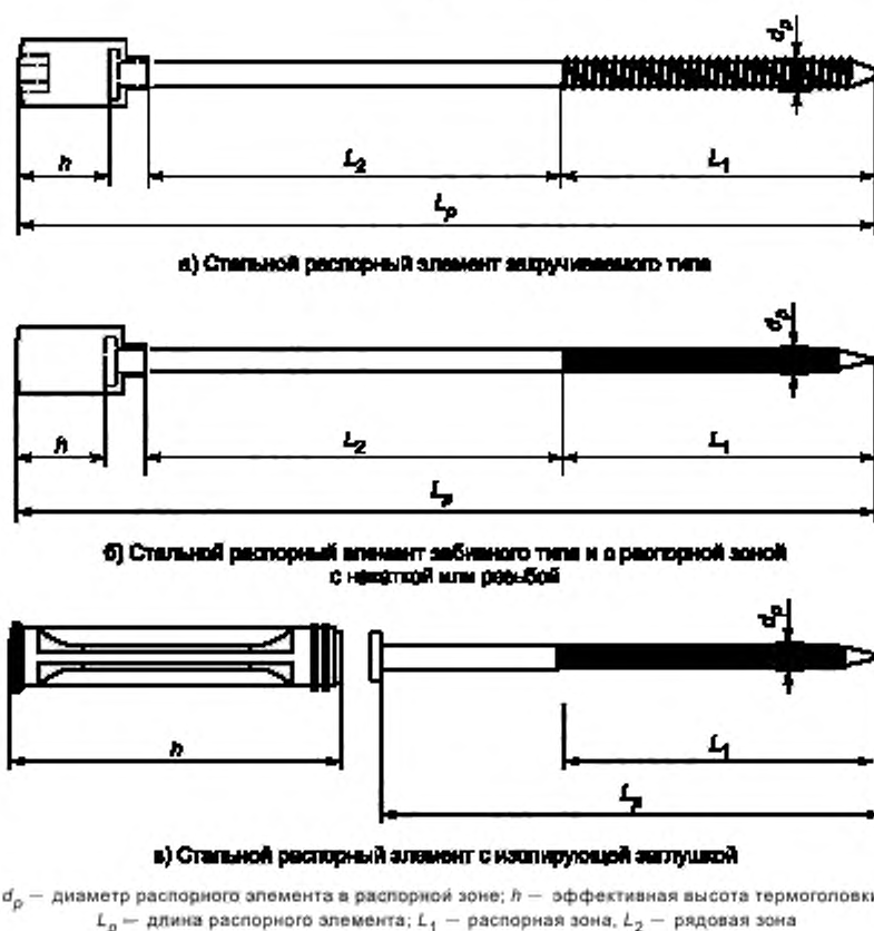
Рисунок 2 — Пример конструкции распорных элементов.
