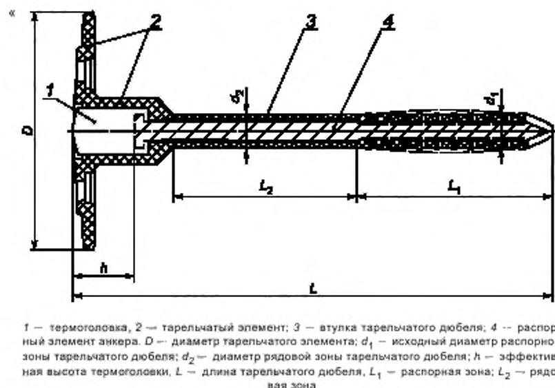
Рисунок 1 — Пример конструкции тарельчатого анкера
