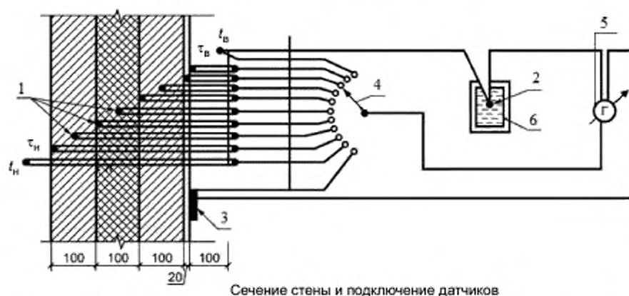
Рисунок А.1 — Схема размещения термопар на испытываемой ограждающей конструкции и подключения их к измерительной аппаратуре
