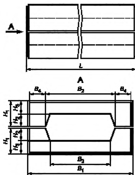
Рисунок А.1 — Форма лотков
