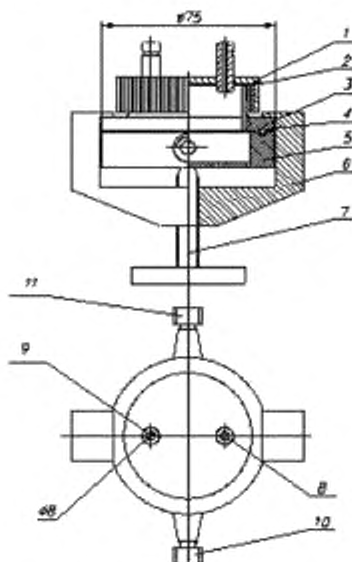
1 — крышка; 2 — прокладка; 3 — диафрагма; 4 — образец материала; 5 — поддон; 6 — трубка; 7 — винт; 8, 9 — штуцера крышки; 10, 11 — штуцера поддона
