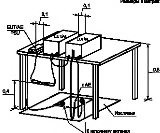
Рисунок D.8 — Пример схемы измерения настольного EUT (измерение излучаемой электромагнитной эмиссии)
