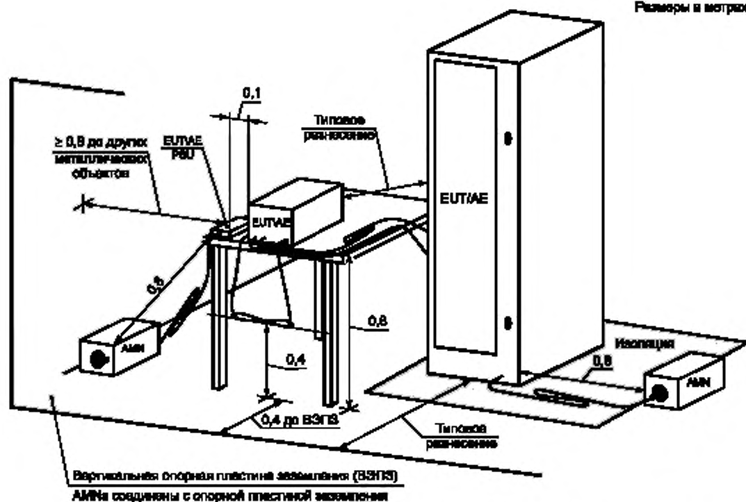
Рисунок D.7 — Пример схемы измерения комбинаций EUT (измерение кондуктивной электромагнитной эмиссии)
