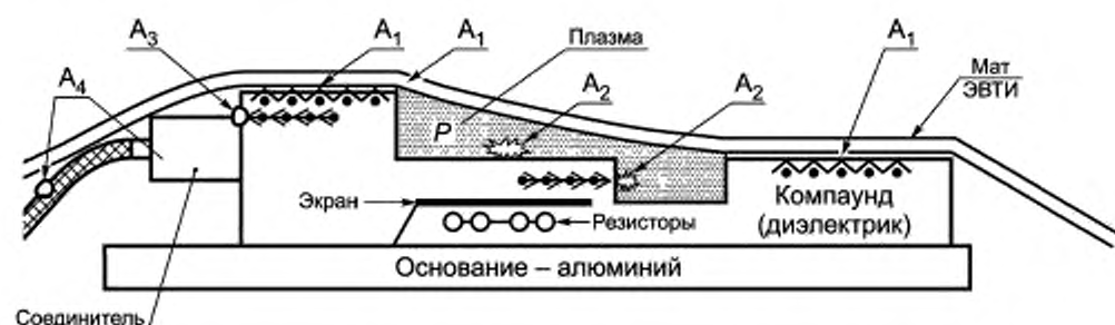
А 1 — пробои с поверхности на пленку ЭВТИ; А 2 — пробои объемного заряда на поверхность изолятора, А 3 — пробой объемного заряда на соединитель кабеля; А 4 — пробой заряда изоляции на оплетку кабеля
