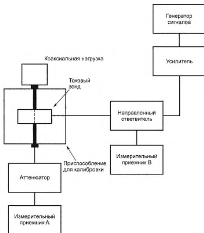
Рисунок М.2 — Блок-схема калибровки
