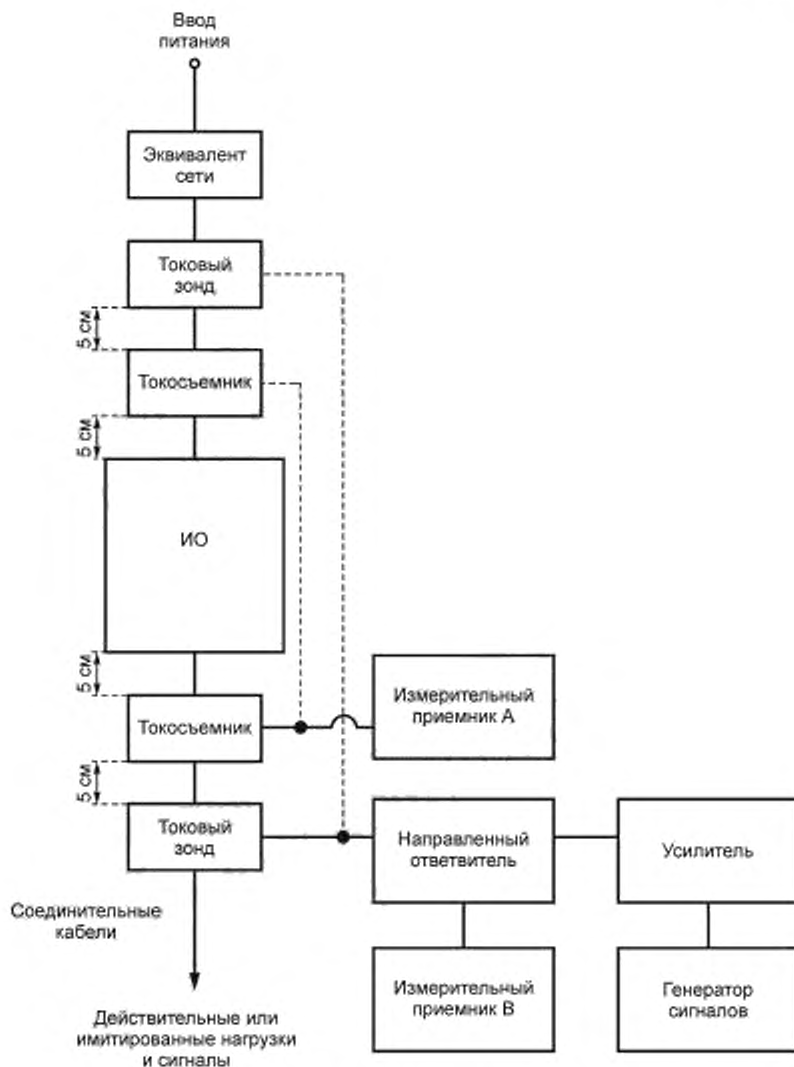
Рисунок М.3 — Блок-схема оценки наводки в кабеле
