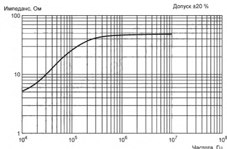
Рисунок В.6 — Импеданс эквивалента сети
