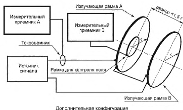
Рисунок Н.1 — Блок-схема калибровки катушек Гельмгольца
