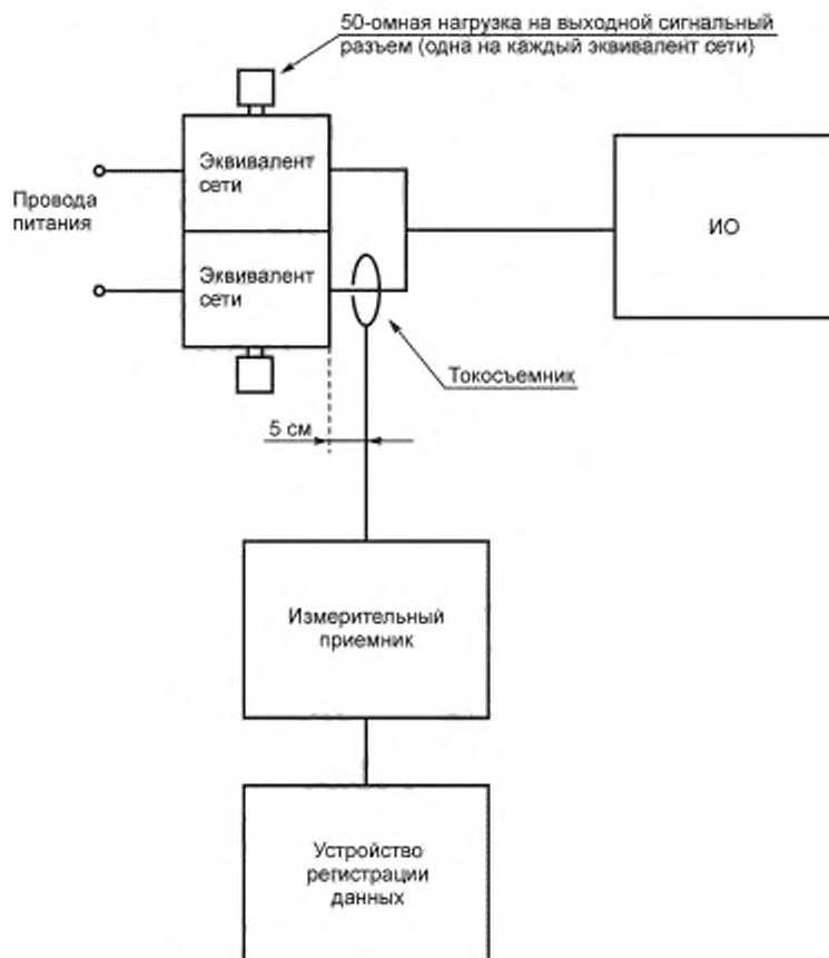
Рисунок В.8 — Блок-схема измерений
