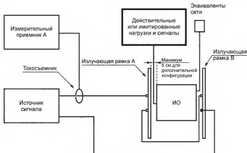
Рисунок Н.2 — Блок-схема испытательной установки с катушками Гельмгольца
