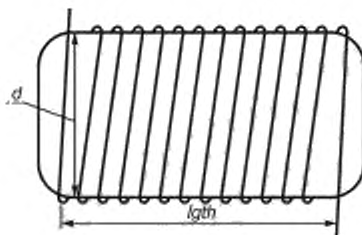
Рисунок Д.1 — Обмотка дросселя
