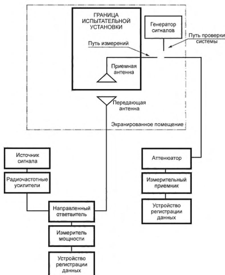
Рисунок П.4 — Метод приемной антенны (1—40 ГГц)
