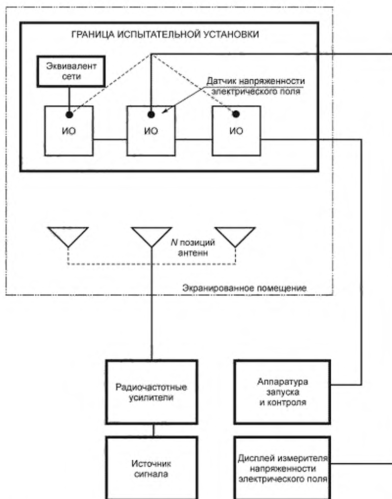
Рисунок П.2 — Несколько позиций испытательных антенн для частоты &gt; 200 МГц
