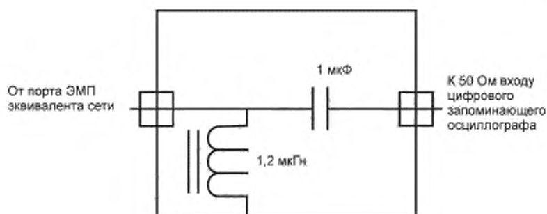
Рисунок Д.4 — Режекторный фильтр частоты питания
