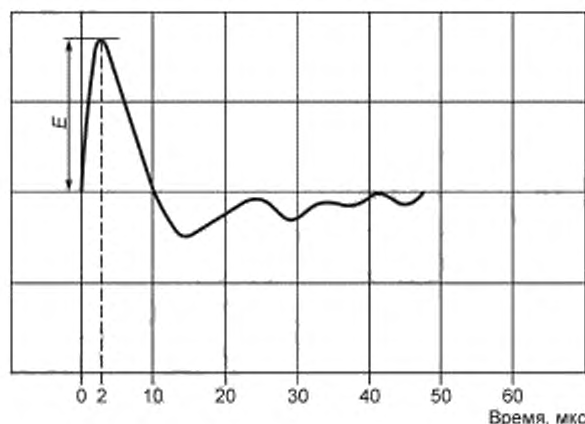
Рисунок Л.1 — Форма импульса напряжения
