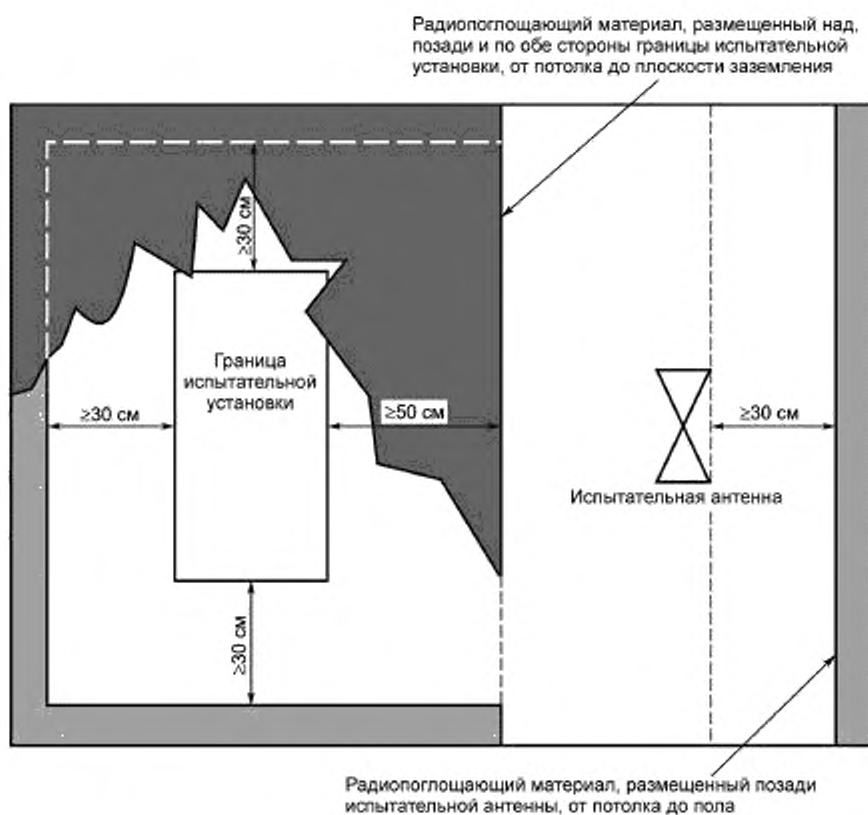
Рисунок И.1 — Схема распределения радиопоглощающего материала
