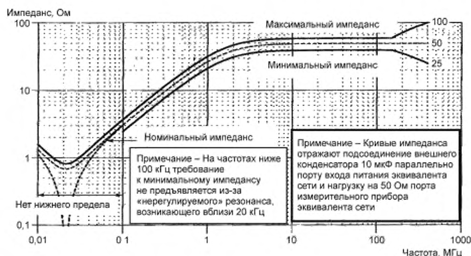
Рисунок Е.1 — Входной импеданс эквивалента сети
