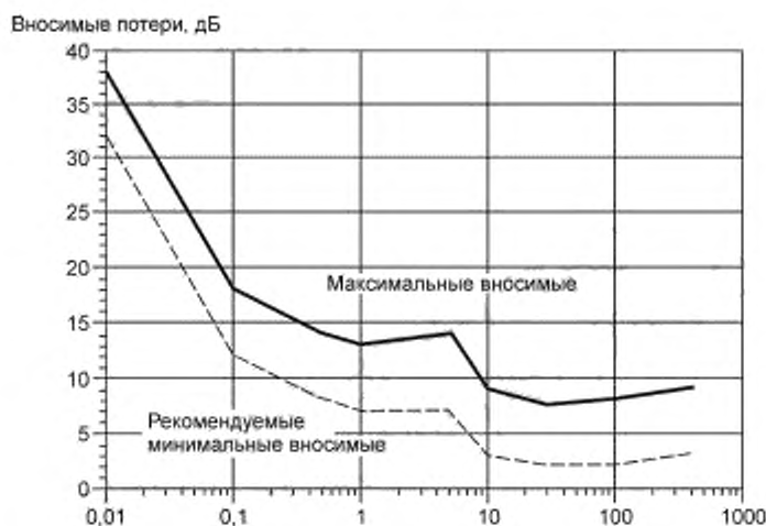
Рисунок Е.2 — Нормы вносимых потерь токового зонда
