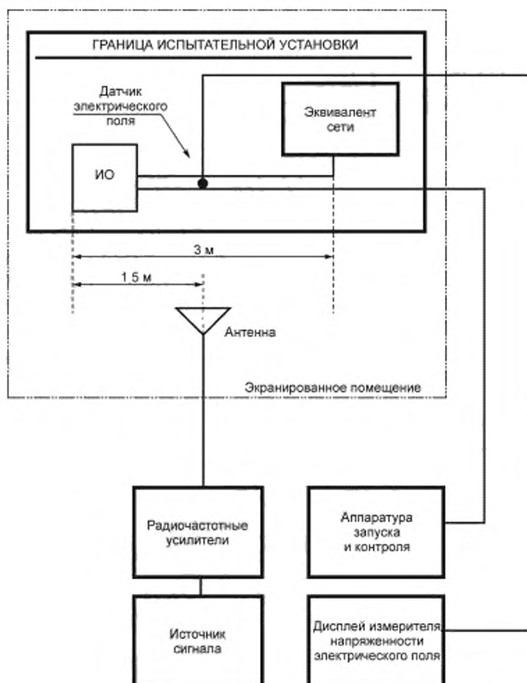
Рисунок П.1 — Блок-схема испытательной установки
