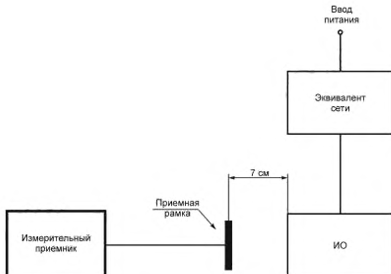
Рисунок Ж.2 — Базовая блок-схема испытаний
