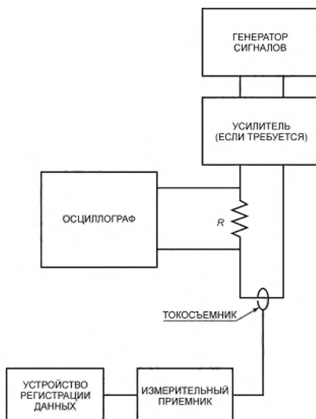
Рисунок В.7 — Блок-схема проверки измерительной системы
