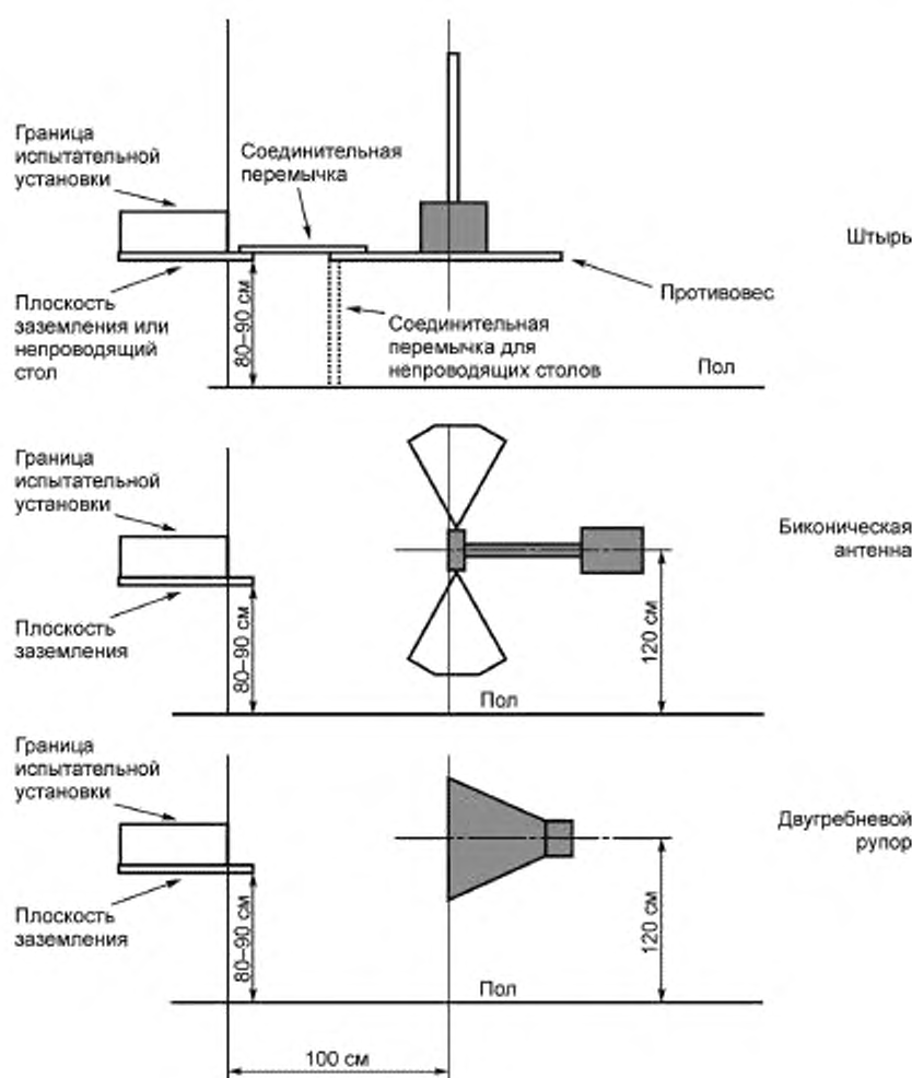
Рисунок И.3 — Установка антенны в заданное положение
