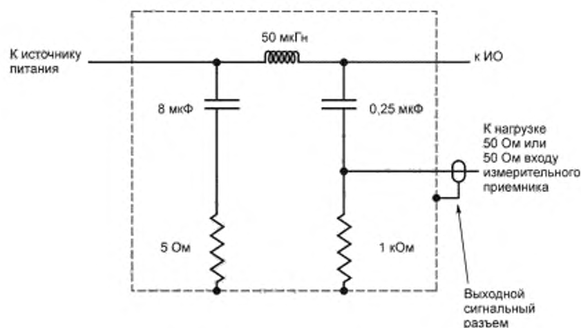
Рисунок В.5 — Схема эквивалента сети
