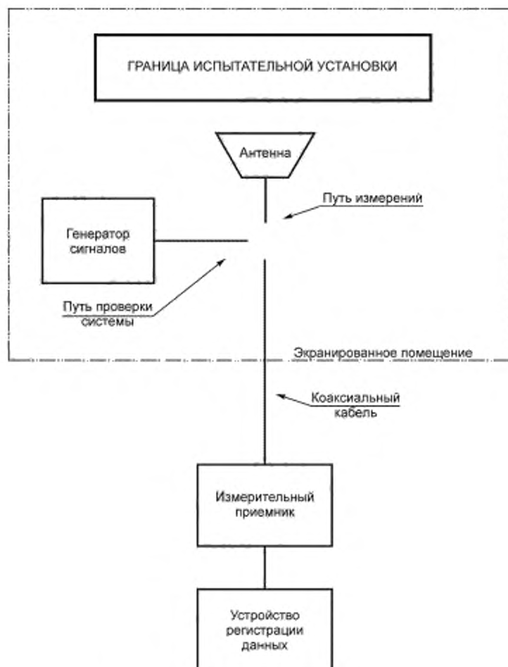
Рисунок И.2 — Базовая блок-схема испытаний
