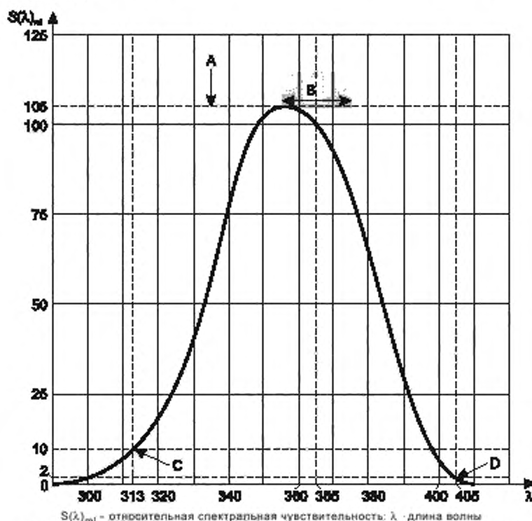
S(\lambda)_{rel} — относительная спектральная чувствительность; \lambda — длина волны Рисунок 1 — Спектральная чувствительность измерителей УФ-А-излучения
