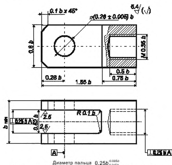
Рисунок В.3 — Рекомендуемая конструкция серег для испытания образцов на внецентренное растяжение.
