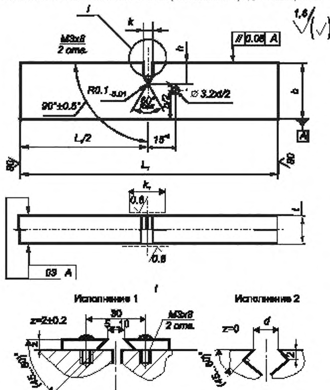
а – образец на трехточечный изгиб
