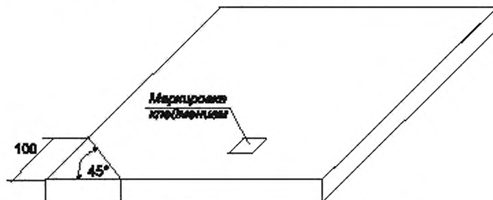
Рисунок Г.1 - Расположение маркировочных полос
