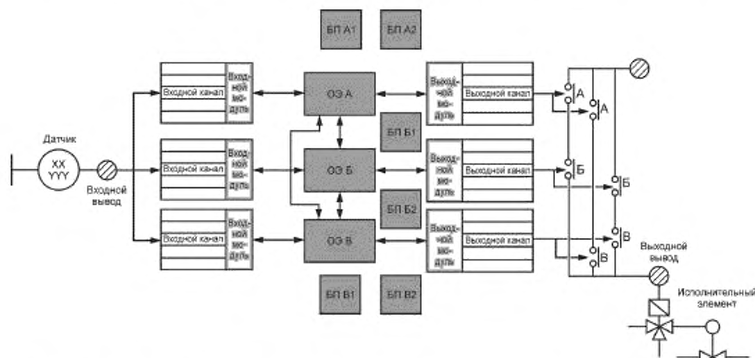
Рисунок В.7 — Три обрабатывающих элемента (ОЗ) с тремя входами/выходами, с межпроцессорной связью и логикой срабатывания 2oo3D
