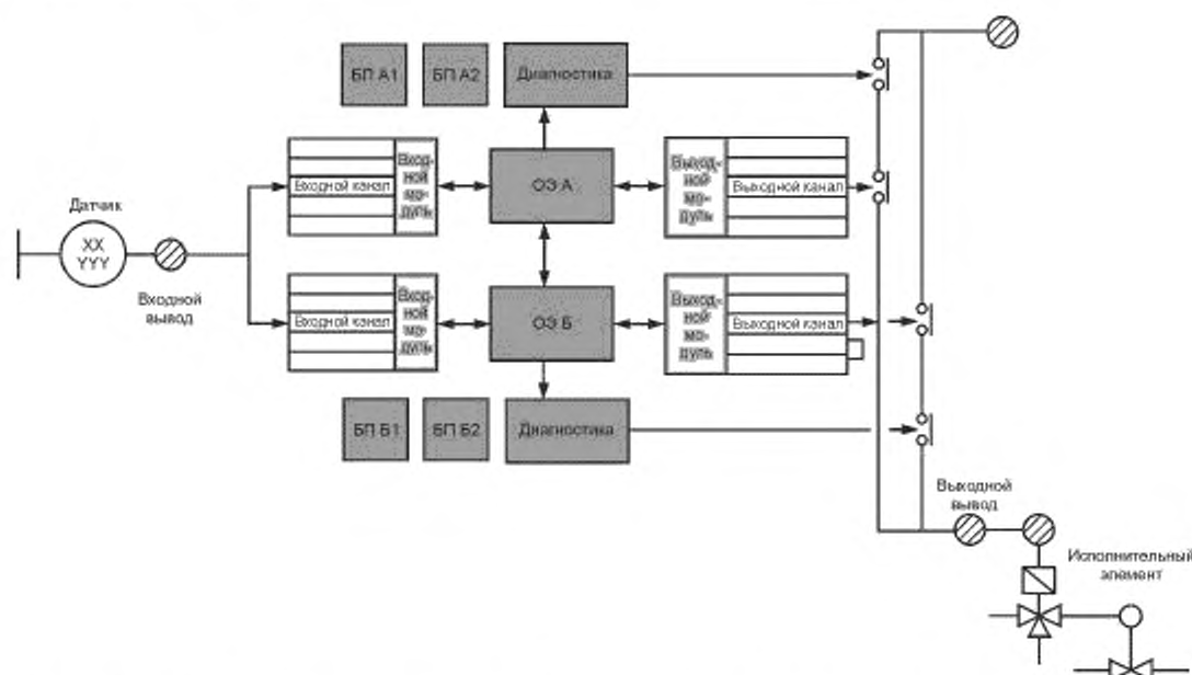
Рисунок В.6 — Два обрабатывающих элемента (ОЗ) с двумя входами/выходами, с межпроцессорной связью, с внешними сторожевыми таймерами и логикой срабатывания 2oo2D
