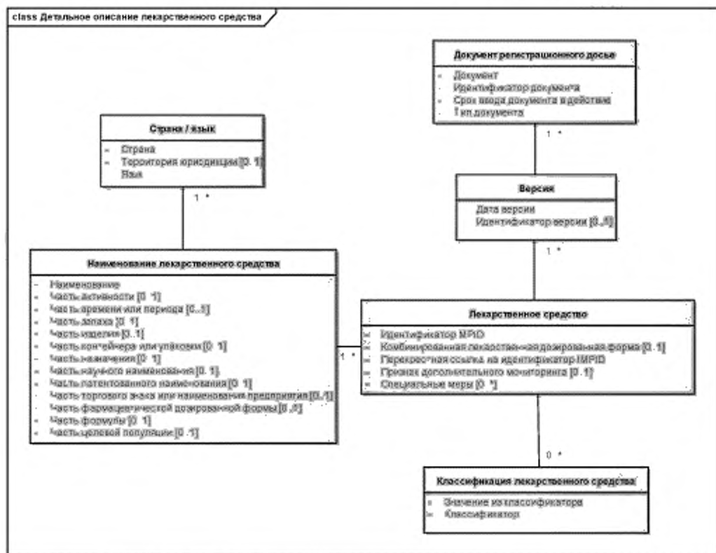
Рисунок 7 — Детальная диаграмма описания раздела лекарственного средства
