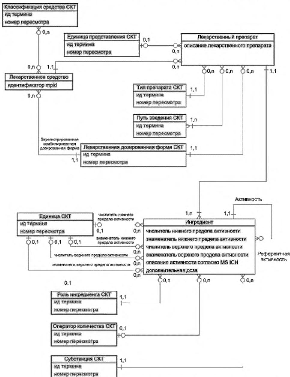
Рисунок G.5 — Пример структуры базы данных описания лекарственного препарата и производенного продукта
