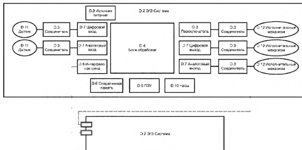
Рисунок D.1 — Общая структура аппаратных средств системы
