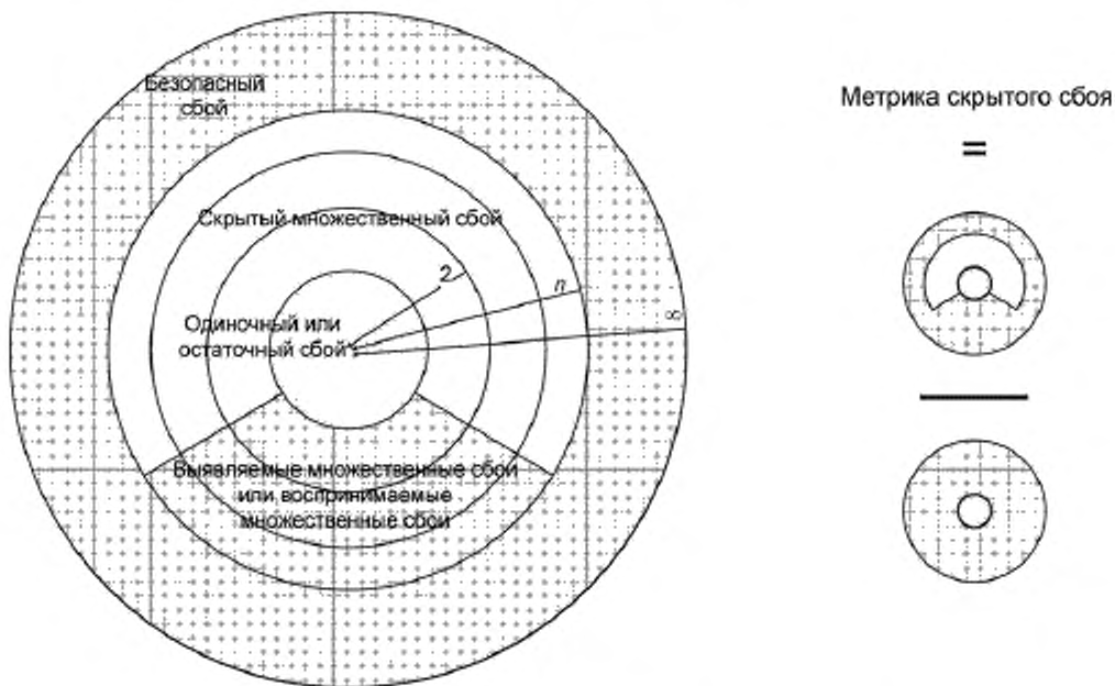
Рисунок С.3 — Графическое представление метрики скрытого сбоя
