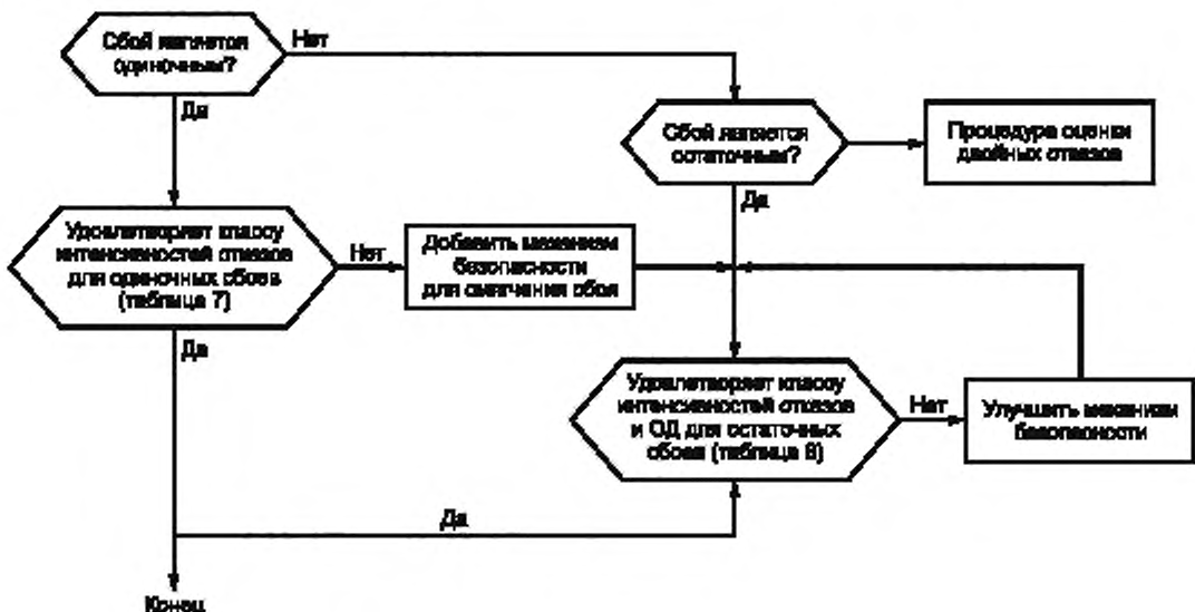
Рисунок 3 — Процедура оценки для одиночных и остаточных сбоев
