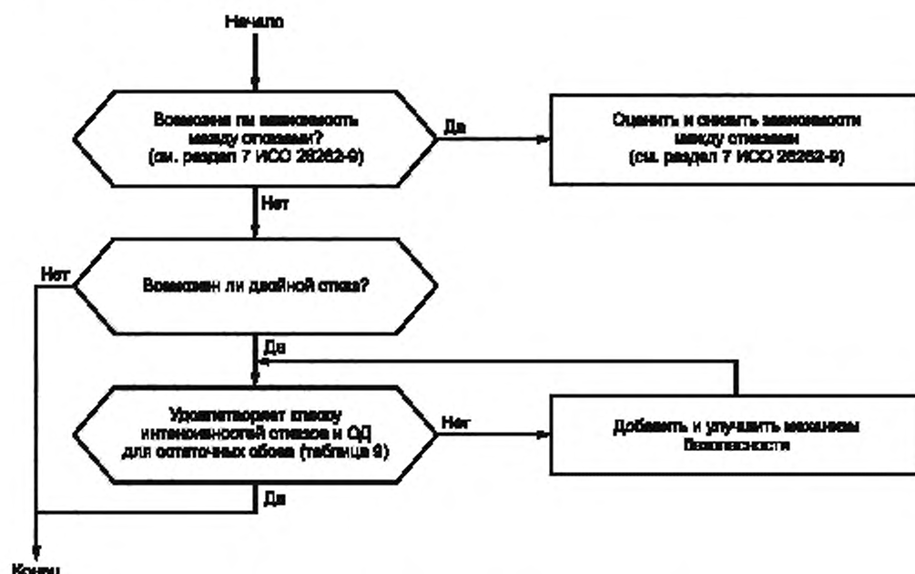
Рисунок 4 — Процедура оценки двойных отказов
