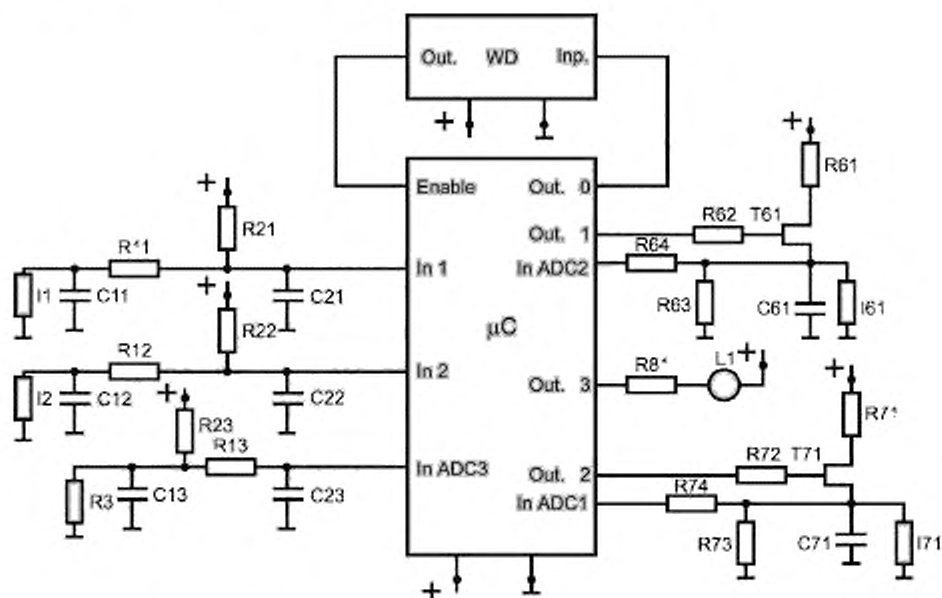
Рисунок Е.1 — Схема рассматриваемого примера
