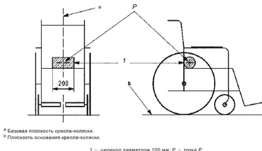
Рисунок 1 — Базовая точка Р кресла-коляски и базовая плоскость кресла-коляски
