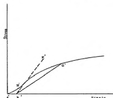
Рисунок A1.2 — Материал с отсутствием линейно-упругой области
