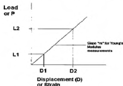
Рисунок X1.1 — Пример кривой модуля для материала
