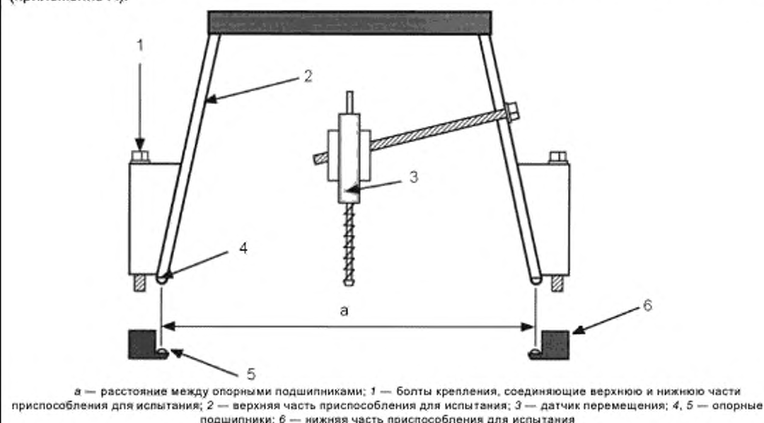
Рисунок 1 — Приспособление для испытания
