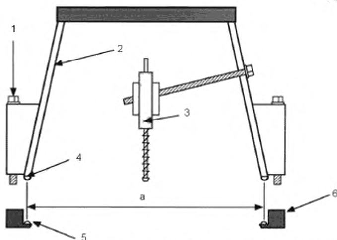
Рисунок 2 — Определение расстояния между опорами для указания размерных допусков образца-панели
