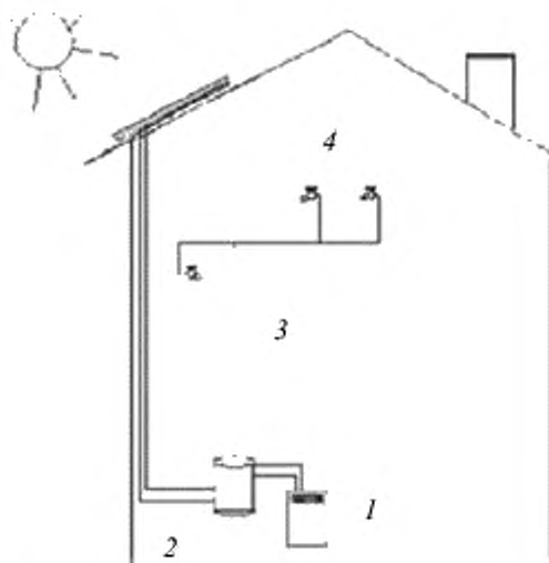
1 – водонагреватель; 2 – накопитель; 3 – система распределения; 4 – водоразбор
