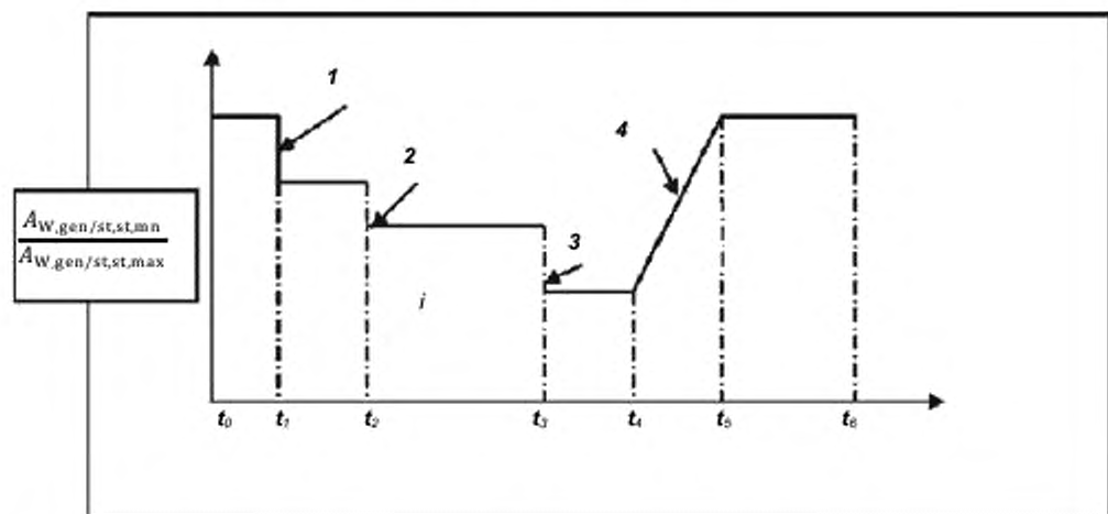
Рисунок Г.1 — Площадь поверхности водонагревателя при водоразборе, используемые для оценки теплопотерь
