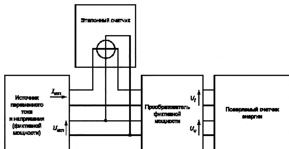
Рисунок А.3 — Схема испытательной цепи с применением источника и преобразователя фигтивной мощности, эталонного ЭЛТА-счетчика с входами «U» и «I» для проверки однофазного ЭЛТА-счетчика
