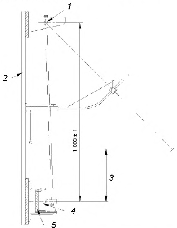
1 — маятник; 2 — основание; 3 — высота падения; 4 — расположение образцов; 5 — установка крепления
