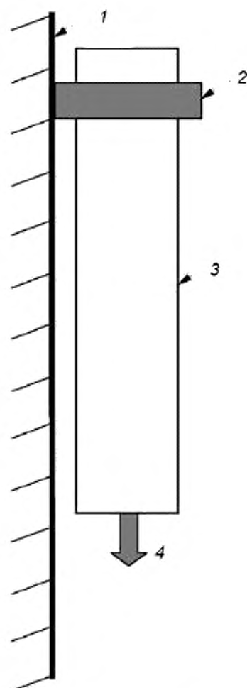
1 — вертикальная монтажная поверхность; 2 — устройство для крепления трубы; 3 — стальная оправка или труба; 4 — груз (включая массу оправки)
