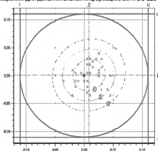
Рисунок 7 – Зона позиционного допуска
