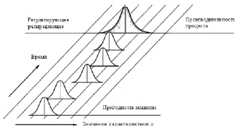
Рисунок 6 – Нестабильный процесс и его пригодность
