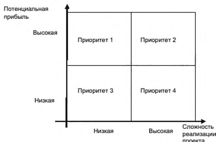
Рисунок 5 — Схема ранжирования
