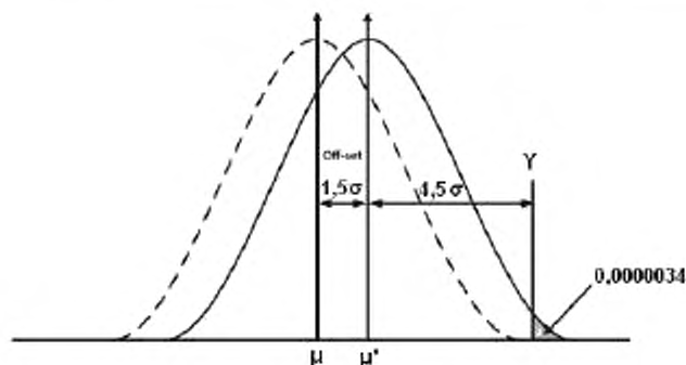
Рисунок 2 — Определение количества сигм
