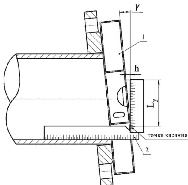
1 — уровень, 2 — угольник
