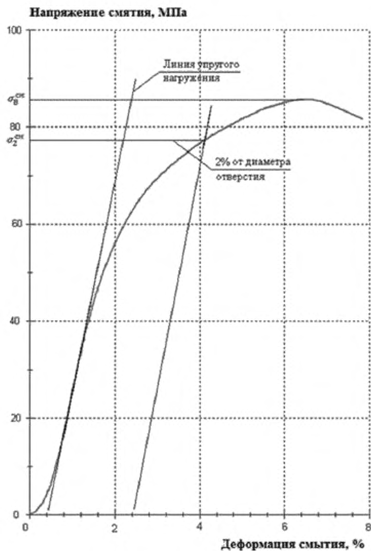
Рисунок 6 — Диаграмма смятия
