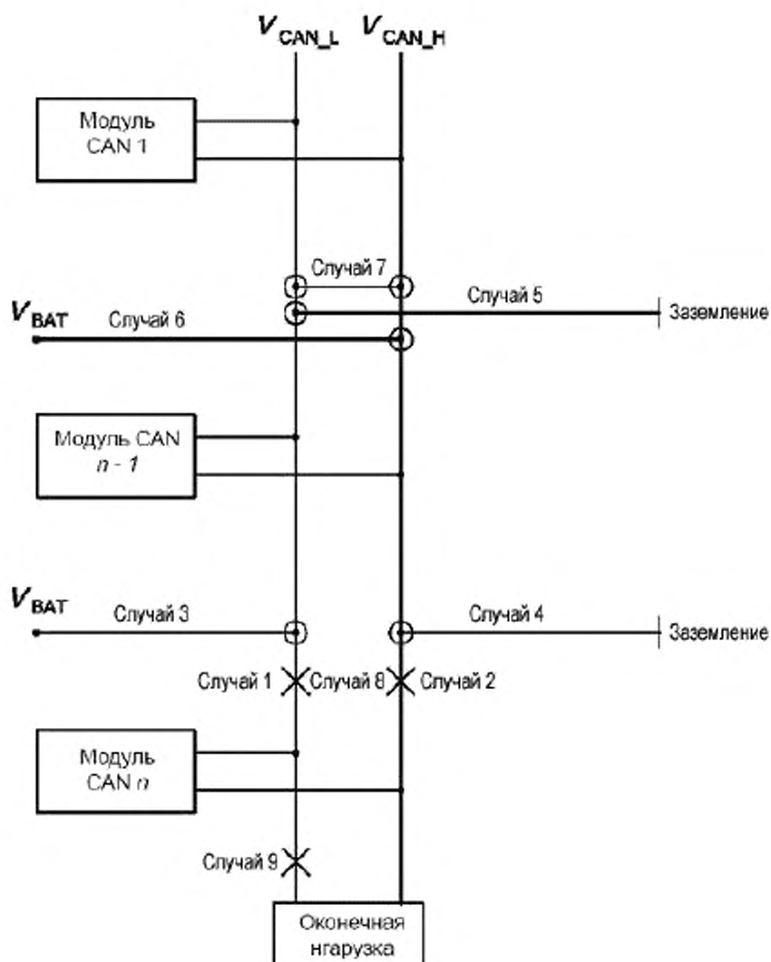
Рисунок 19 — Возможные отказы линий шины
