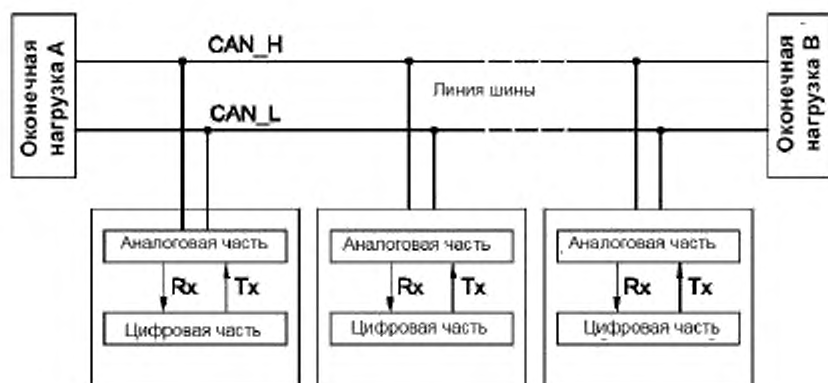
Рисунок 1 — Рекомендуемое электрическое подключение
