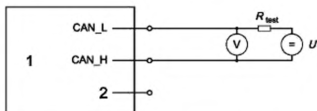
1 — узел CAN со схемой оконечной нагрузки; 2 — заземление
