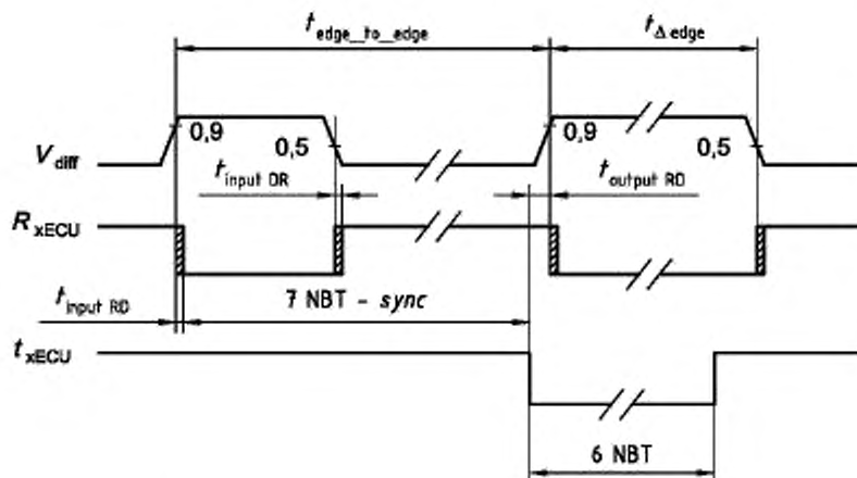
Рисунок 12 — Измерение времени внутренней задержки ECU
