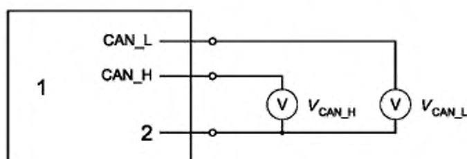
Рисунок 4 — Измерение V_{CAN\_L} и V_{CAN\_H} при свободном состоянии шины
