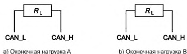
Рисунок 14 — Оконечная нагрузка для высокоскоростной реализации шины
