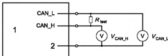
1 — узел CAN со схемой оконечной нагрузки; 2 — заземление
