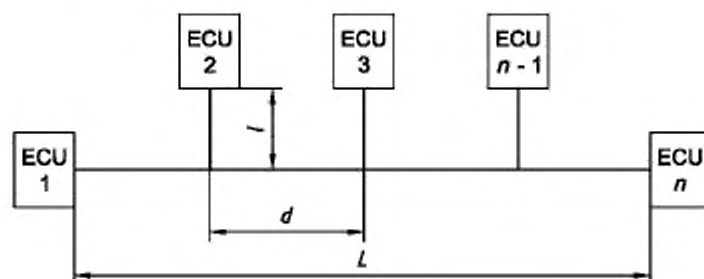
Рисунок 3 — Топология проводки сети
