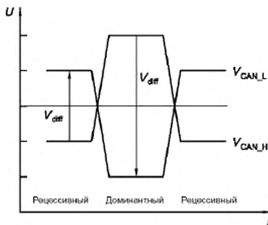
Рисунок 2 — Физическое представление битов
