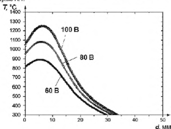
Рисунок А.1 — График зависимости значений температур поверхности нагревателя от значений приложенного электрического напряжения (на осях X и Y) [13]
