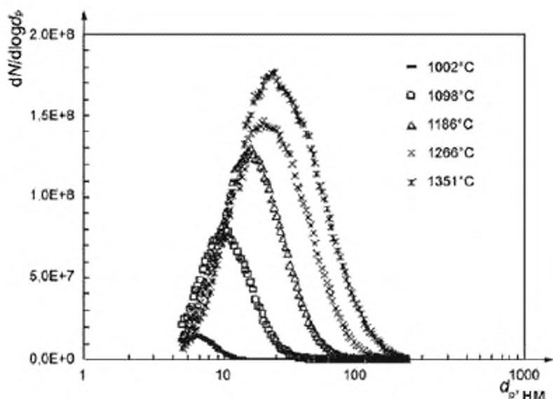
Рисунок А.4 — График зависимости значений распределения наночастиц по размерам от значений температур поверхности нагревателя [13]
