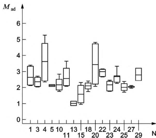
Рисунок А.1 — Отклонение результатов испытаний между лабораториями. Измельченные шины
