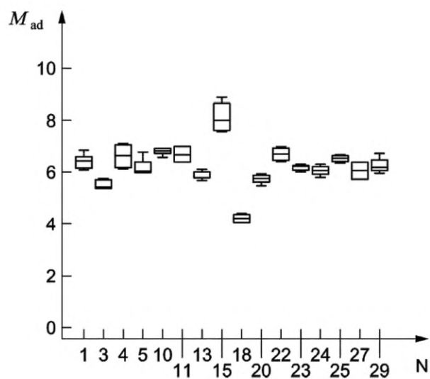
Рисунок А.4 — Отклонение результатов испытаний между лабораториями. Бытовые отходы
