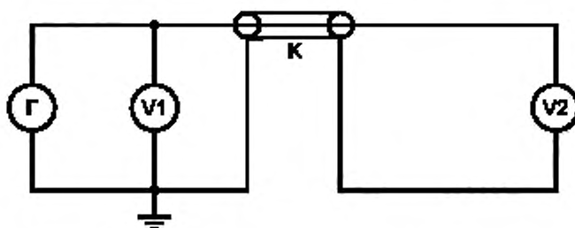
Г — генератор; V1, V2 — вольтметры; К — кабель
