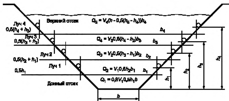
Рисунок 3 — Пример расчета расхода методом послойных сечений
