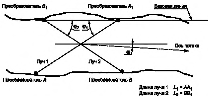
Рисунок 1 — Схема расположения преобразователей с пересекающимися лучами
