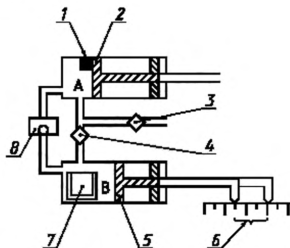
1 — зажим клапана; 2 — снабжающий поршень; 3 — клапан, восстанавливающий равновесие в давлении; 4 — соединительный клапан; 5 — измерительный поршень; 6 — изменение объема; 7 — стакан для пробы; 8 — прибор для измерения разницы давления
