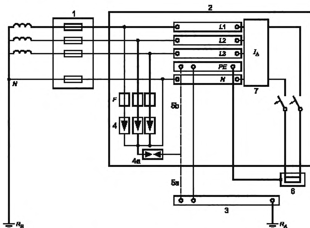
1 — ввод распределительной сети; 2 — распределительный щит; 3 — главный заземляющий зажим (шина); 4 — УЗИП; 4а — УЗИП по 534.2.3.2 или искровой разрядник; 5а, 5б — заземление УЗИП; 6 — защищаемое оборудование; 7 — УДТ; F — защитное устройство, указанное изготовителем (предохранитель, автоматический выключатель, УДП); R_A — заземляющий электрод (сопротивление); R_B — заземляющий электрод (сопротивление) системы питания
