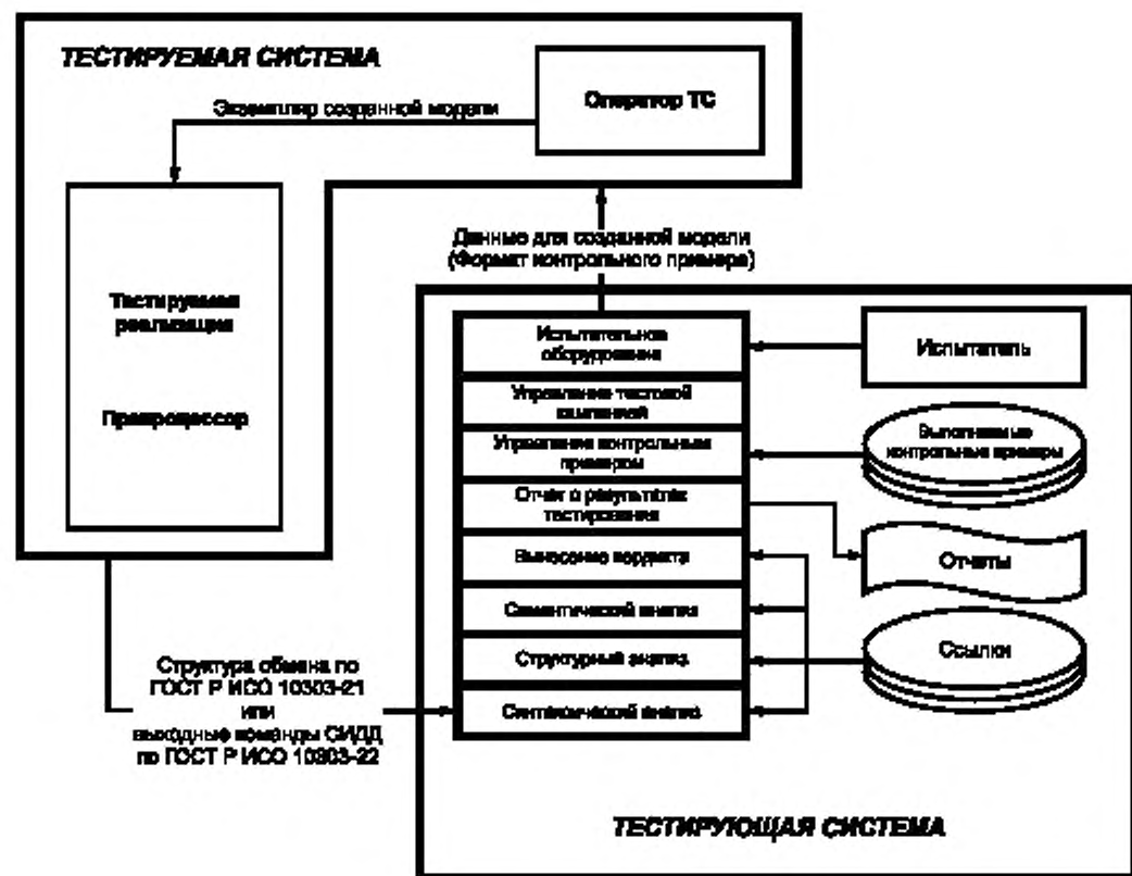
Рисунок 1 — Компоненты тестирования препроцессора
