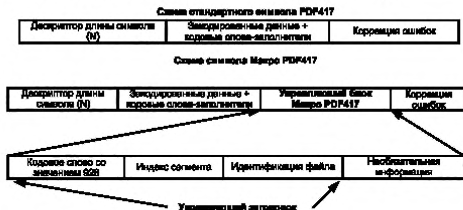
Рисунок Н.1 — Схемы символов PDF417
