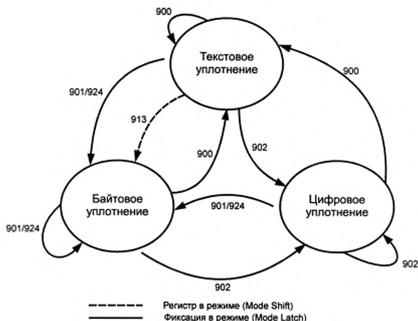
Рисунок 5 — Возможные переходы между режимами.
