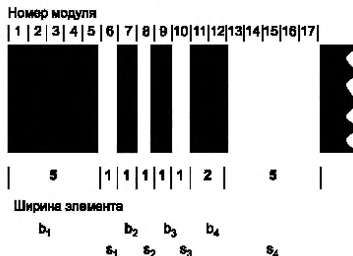
Рисунок 3 — Знак символа PDF417.
