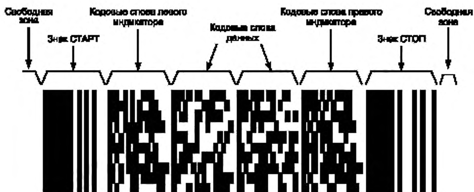
Рисунок 1 — Структура символа PDF417.
