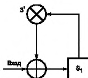
Рисунок L.1 — Делитель синдрома символа
