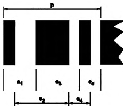
Рисунок К.1 — Размеры для декодирования
