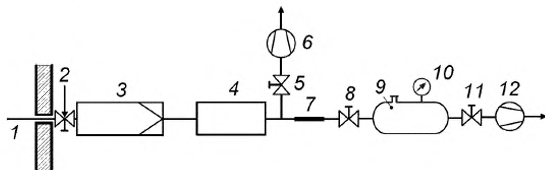
1 — зонд для отбора проб подогреваемый (при необходимости); 2 — вентиль для ввода контрольных газов; 3 — фильтр для улавливания твердых частиц, подогреваемый; 4 — блок охлаждения и осушки пробы газа; 5 — регулирующий вентиль; 6 — побудитель расхода газа; 7 — дроссель; 8 — запорный вентиль; 9 — сосуд или канистра для отбора проб; 10 — средства измерений температуры и давления; 11 — запорный вентиль; 12 — вакуумный насос (при необходимости)
