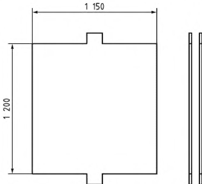
Рисунок D.2 – Эскиз разобранной емкости для проб
