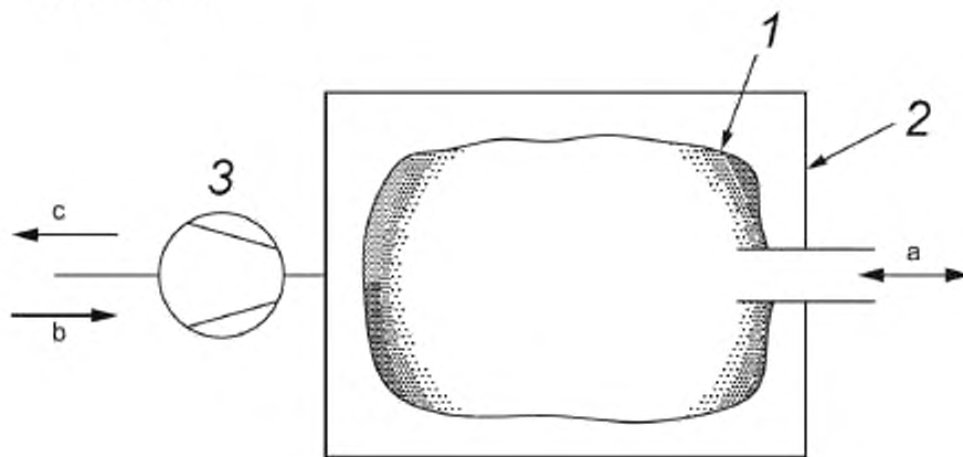
1 — емкость для проб; 2 — корпус емкости для проб; 3 — вентилятор; a — отбираемая или подаваемая проба воздуха; b — выпуск воздуха; c — заполнение воздухом
