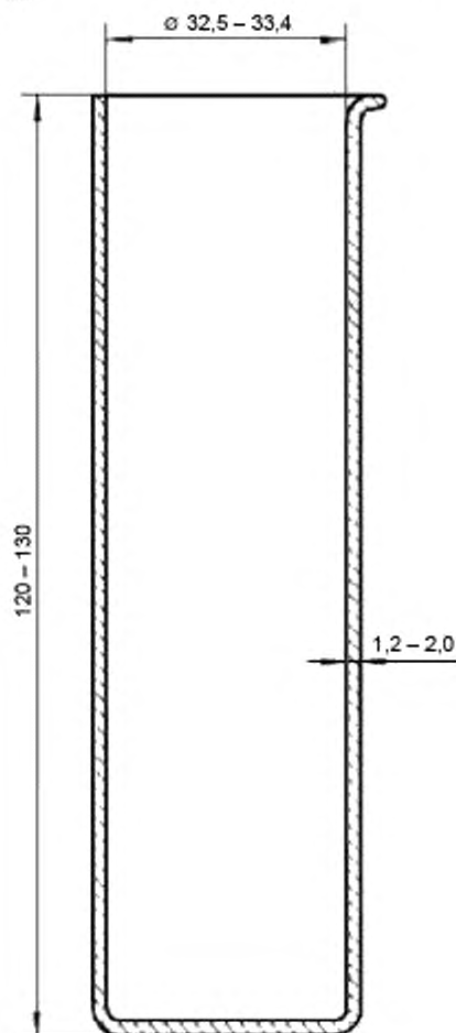
Рисунок 1 – Стеклянный сосуд для образца
