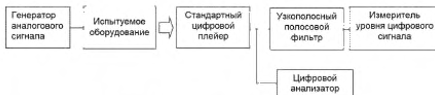
Рисунок 28 — Схема соединения оборудования
