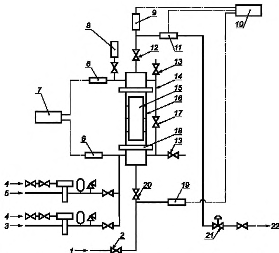
1 — источник газа или воды под высоким давлением; 2 — клапан-регулятор потока; 3 — источник газа для испытаний; 4 — подача воздуха; 5 — источник испытательной жидкости; 6 — средство измерения давления; 7 — регистрирующее устройство; 8 — расходомер для азота; 9 — устройство измерения выходного давления; 10 — диаграммный самописец; 11 — расходомер; 12 — выпускной запорный клапан; 13 — спусной клапан; 14 — уравнительная линия; 15 — SSSV; 16 — испытательная секция; 17 — уравнительный клапан; 18 — соединитель; 19 — средство измерения давления на входе; 20 — впускной запорный клапан; 21 — регулятор давления на выходе; 22 — возврат воды или газа
