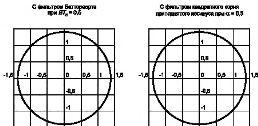
Рисунок 6 — Фазовые диаграммы для модуляции QPSK с применением разных типов фильтров
