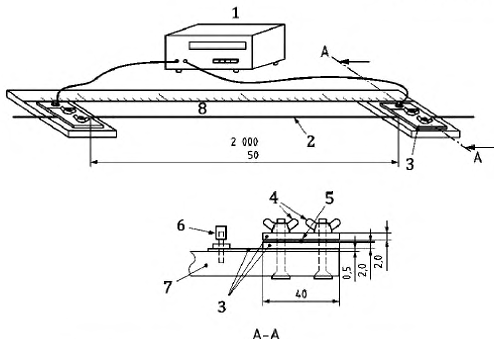
1 — измеритель сопротивления; 2 — образец для испытаний; 3 — электрод (медный); 4 — скрепляющая гайка; 5 — образец для испытаний; 6 — вывод (контакт); 7 — изолирующая пластина; 8 — измеритель длины
