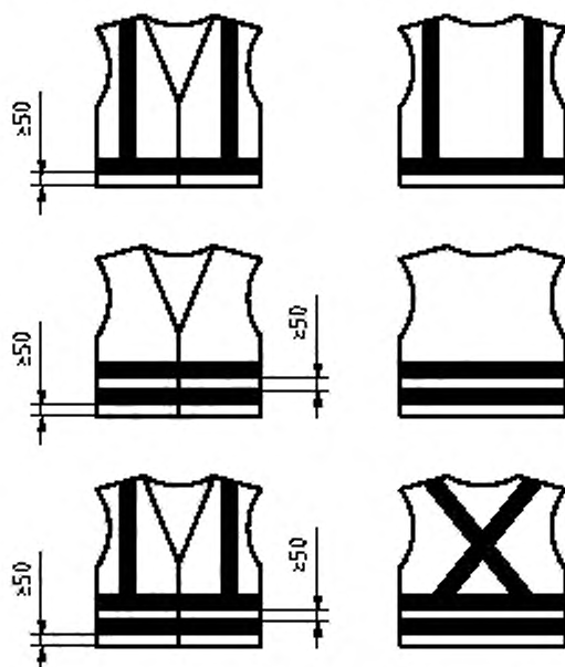
Рисунок 1 — Примеры предметов одежды, покрывающей только туловище
