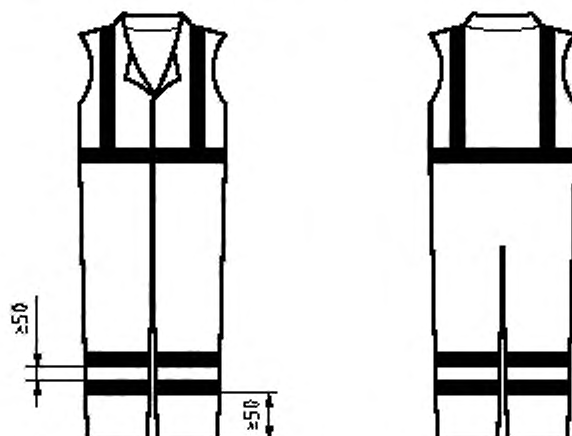
Рисунок 4 — Пример одежды, покрывающей туловище и ноги
