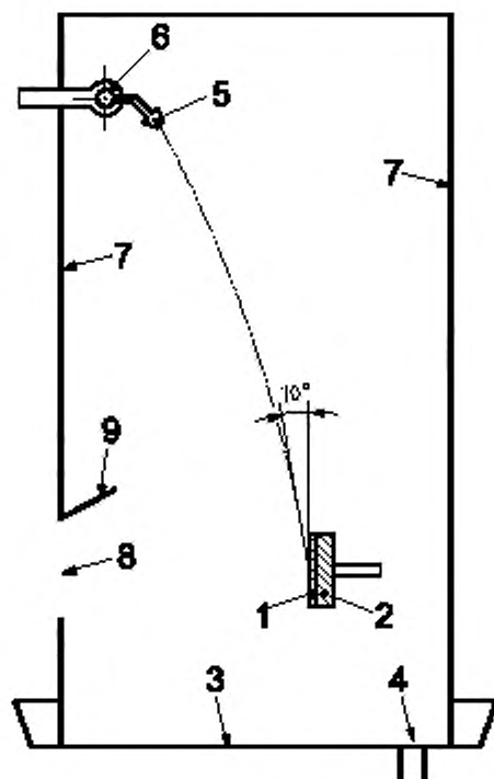
1 — образец; 2 — держатель; 3 — лоток для сбора воды; 4 — дренажная труба; 5 — форсунка; 6 — гибкое соединение; 7 — кожух; 8 — отверстие; 9 — водосточный желоб
