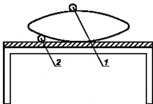
Рисунок 4 — Подушки/валики: положение источника возгорания
