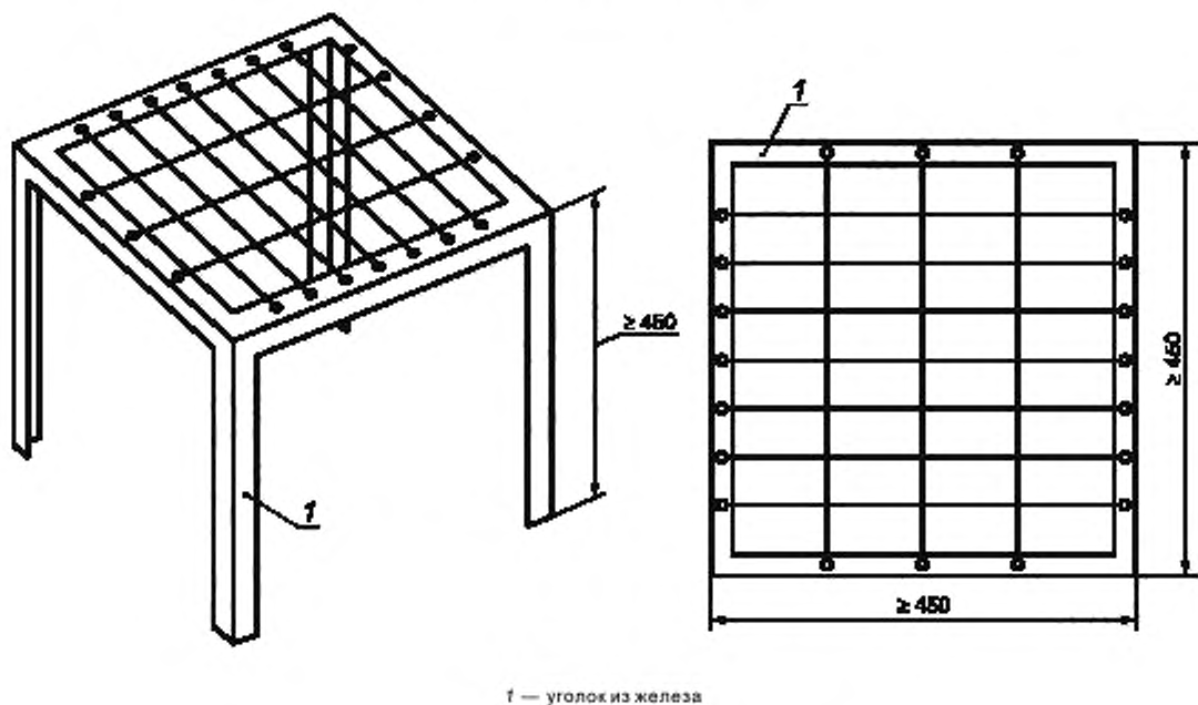
Рисунок 1 — Пример испытательного стенда
