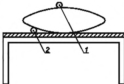
Рисунок 5 — Подушки/валики: расположение сигарет
