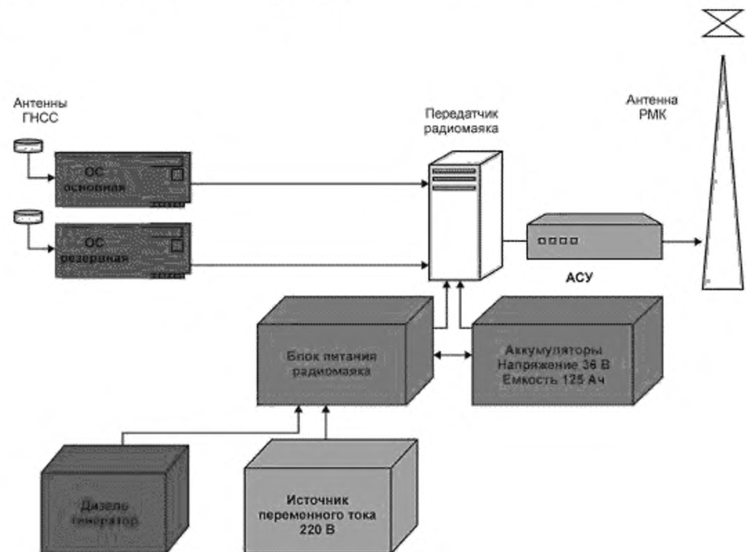
Рисунок 3 — Схема межблочных соединений и питания радиомаяка
