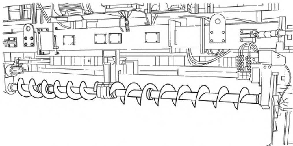
Рисунок А.7 — Типовой распределительный шнек бетоноукладчика
