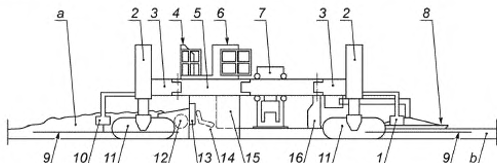
1 — датчик уровня и курса, задний; 2 — выравнивающий цилиндр; 3 — шарнирная стойка; 4 — платформа оператора; 5 — основная рама; 6 — силовой агрегат; 7 — механизм для укладки арматурных стержней; 8 — отделочный брус; 9 — копирная струна; 10 — датчики уровня и курса, передние; 11 — гусеничная тележка в сборе; 12 — распределительный шнек; 13 — передний дозирующий разравнивающий брус; 14 — высокочастотные вибраторы; 15 — экструзионный поддон; 16 — плавающий поперечный отделочный брус; а — выгруженная бетонная смесь; б — готовая бетонная плита
