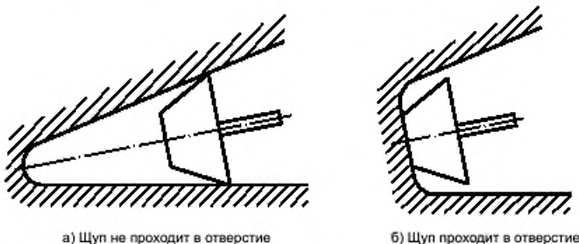
Рисунок A.4 — Примеры проведения испытаний V-образных отверстий на застревание
