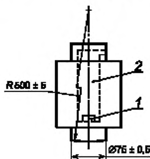
1 — датчик ускорения; 2 — место установки датчика ускорения
