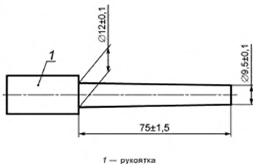
Рисунок Г.1 — Размеры испытательного штифта
