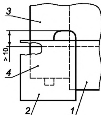
1 — платформа для ног (может быть внахлест с полотном); 2 — защитный кожух; 3 — беговое полотно; 4 — задний ролик
